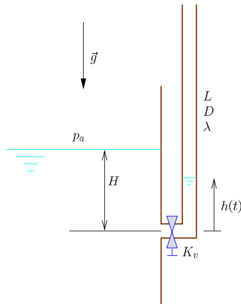
Figura 21.19: Descarga por un tubo vertical con codo y válvula.
