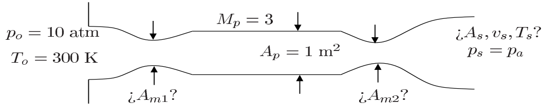
Figura 18.23: Túnel aerodinámico
