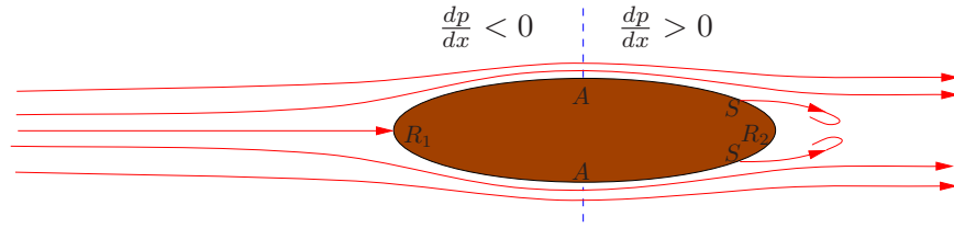
Figura 19.3: Flujo alrededor de un cuerpo sólido.
