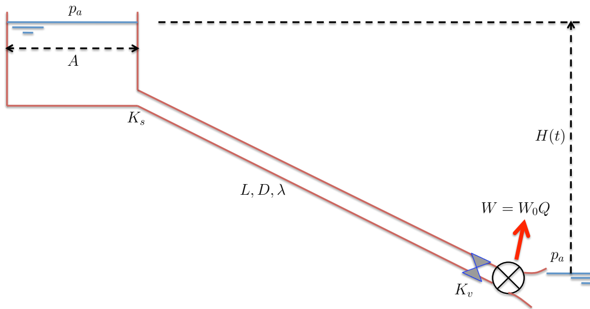
Figura 21.29: Miniturbina.
