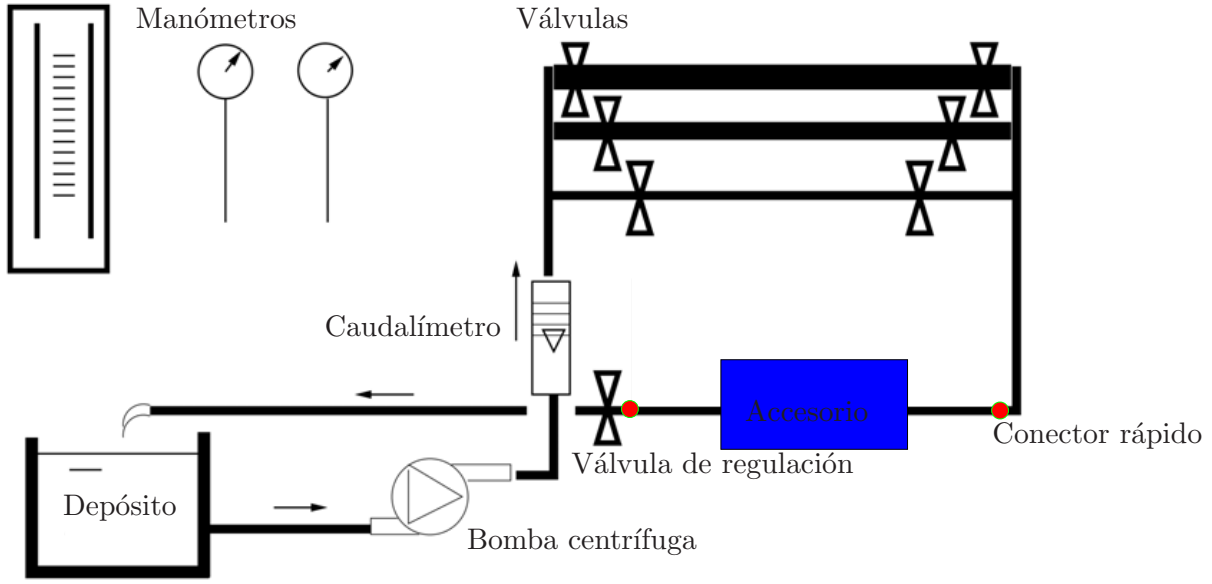
Figura 21.30: Esquema de la instalación.
