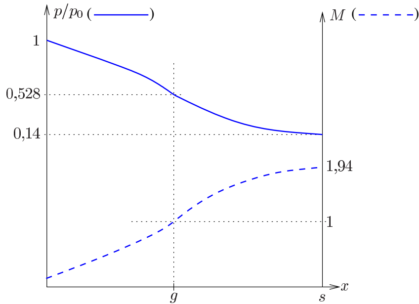
Figura 18.5: Flujo supersónico
