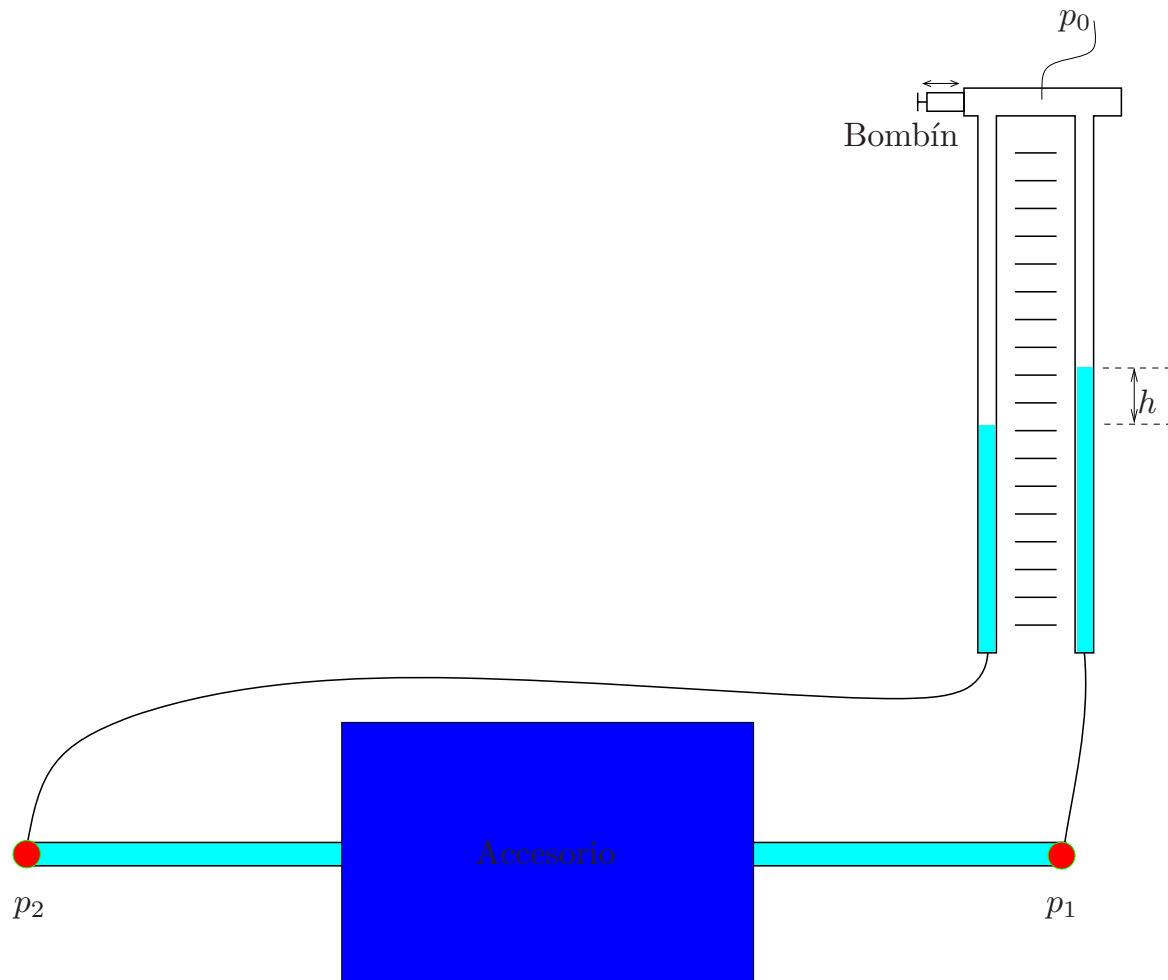
Figura 21.31: Manómetro diferencial.
