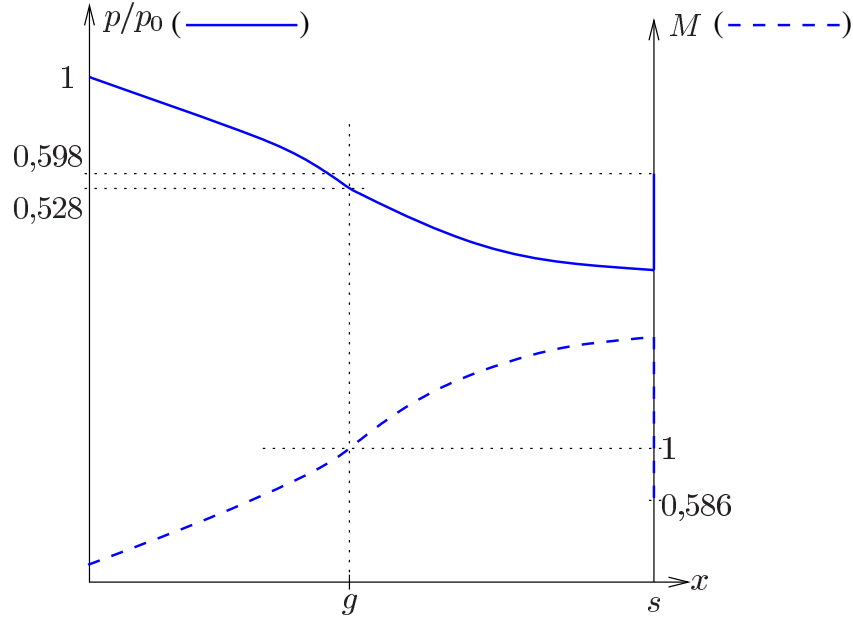
Figura 18.6: Flujo supersónico
