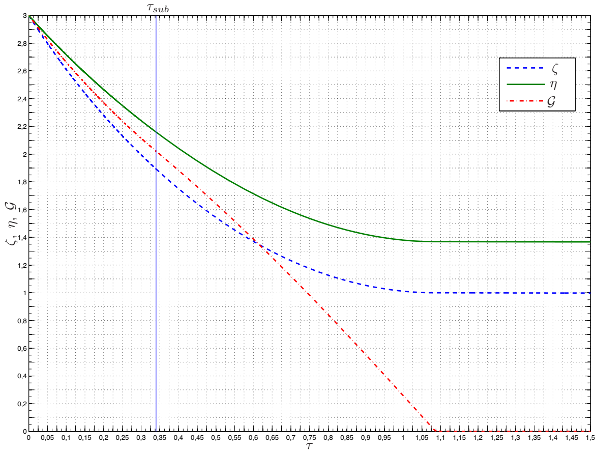
Figura 18.27: Evolución de las magnitudes adimensionales \eta , \zeta y \mathcal{G} frente a \tau para k = 3 , T_a = 20 °C y \gamma = 1,4 .
