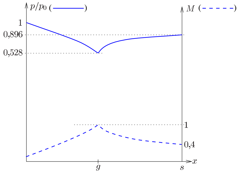
Figura 18.4: Flujo subsónico
