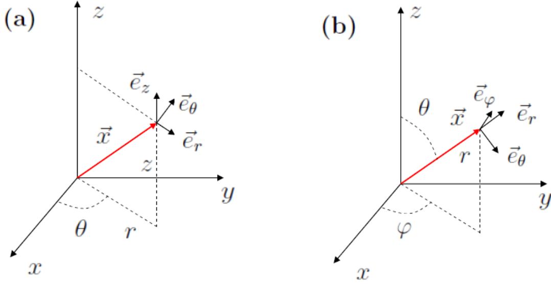
Figura 2.6: (a) Coordenadas cilíndricas. (b) Coordenadas esféricas.
