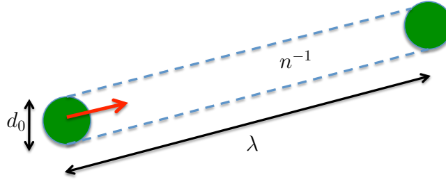
Figura 8.2: Camino libre medio entre colisiones.
