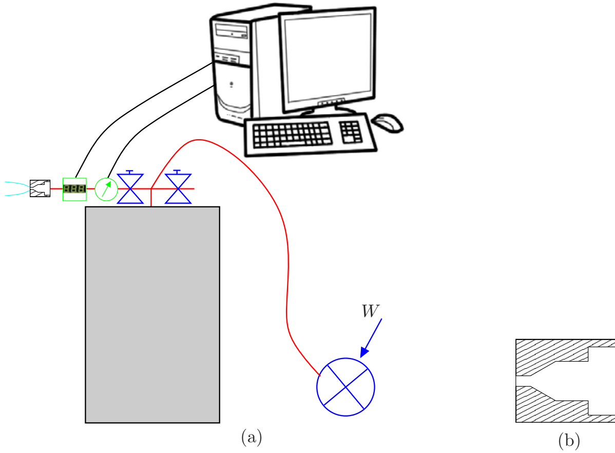
Figura 18.26: (a) Esquema de la instalación. (b) Ampliación de la sección longitudinal de la tobera convergente (el diámetro de salida es de 1 mm).
